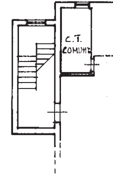
PIANTA PIANO SEMINTERRATO
