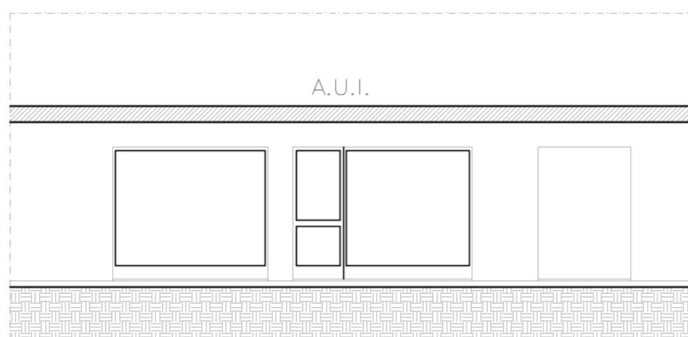
PROSPETTO FRONTALE VISTA DA SOTTO IL PORTICATO STATO DI FATTO
