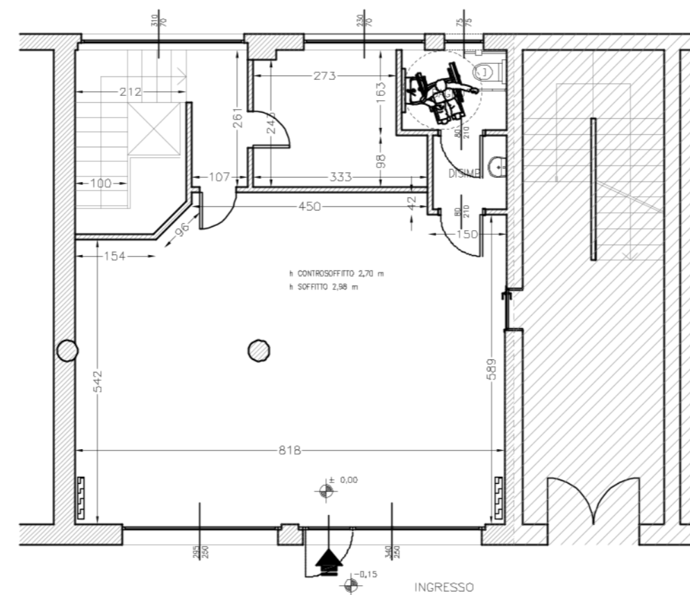
PIANO TERRA STATO DI FATTO
