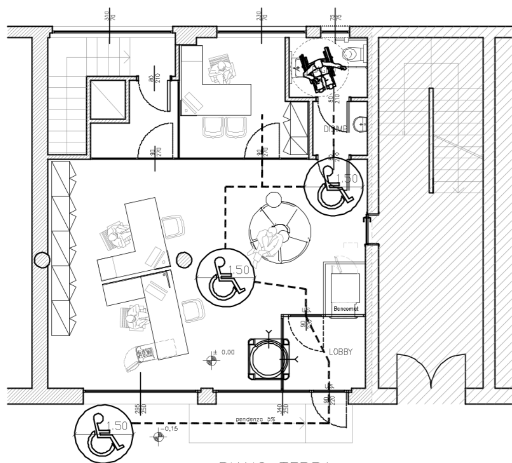
PIANO TERRA VERIFICA REQUISITO DI VISITABILITA'
