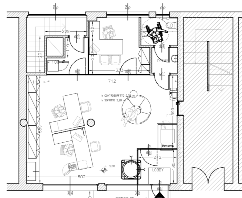
PIANO TERRA PROGETTO
