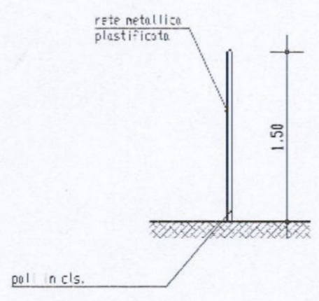
SEZIONE B - B SCALA 1:50
