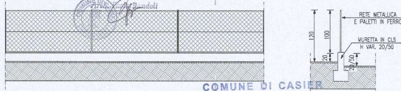
Prospetto nuova recinzione Scala 1/50
