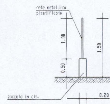
SEZIONE C - C SCALA 1:50
