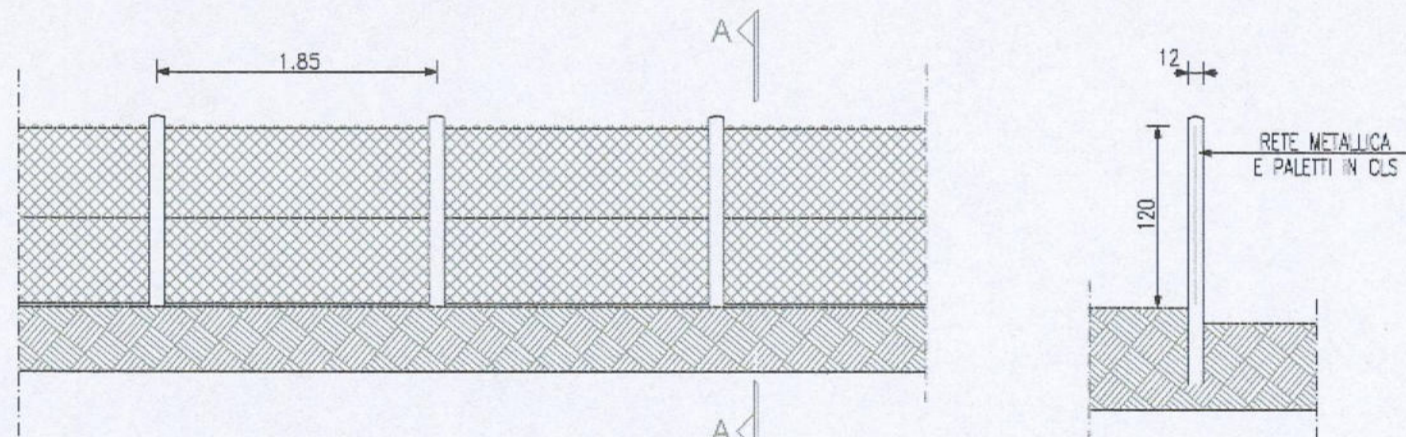
COMMISSIONE COMUNALE EDILIZIA Prospetto recinzione esistente Scala 1/50
