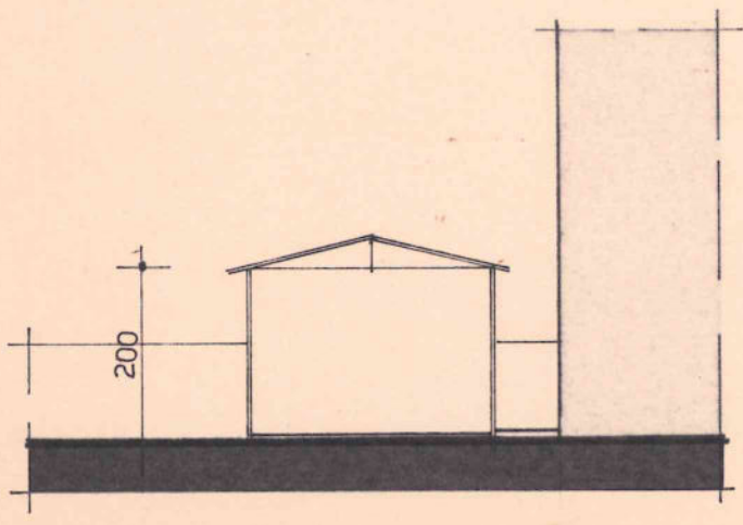
SEZIONE D-D
