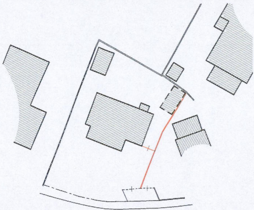
PLANIMETRIA Scala 1/500
