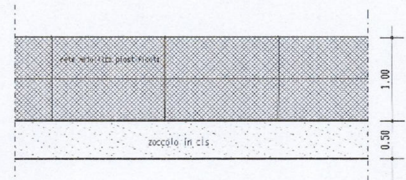
PROSPETTO SCALA 1:50
