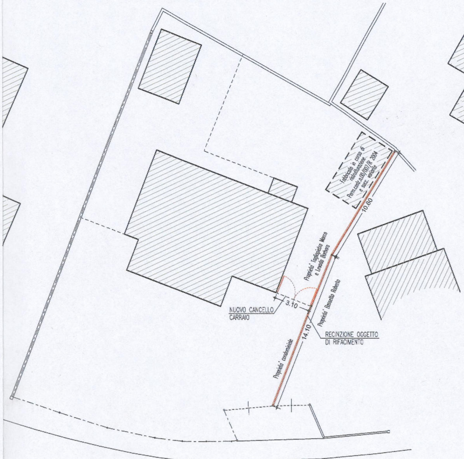
PLANIMETRIA Scala 1/200
