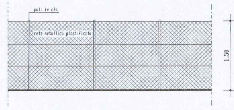
PROSPETTO SCALA 1:50
