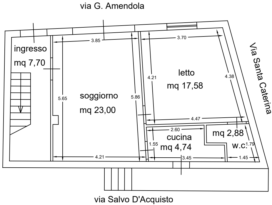
Pianta Piano Terra h= 3,50
