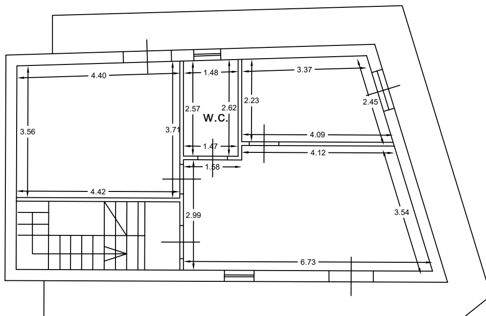
Pianta Piano Primo h= 3,20
