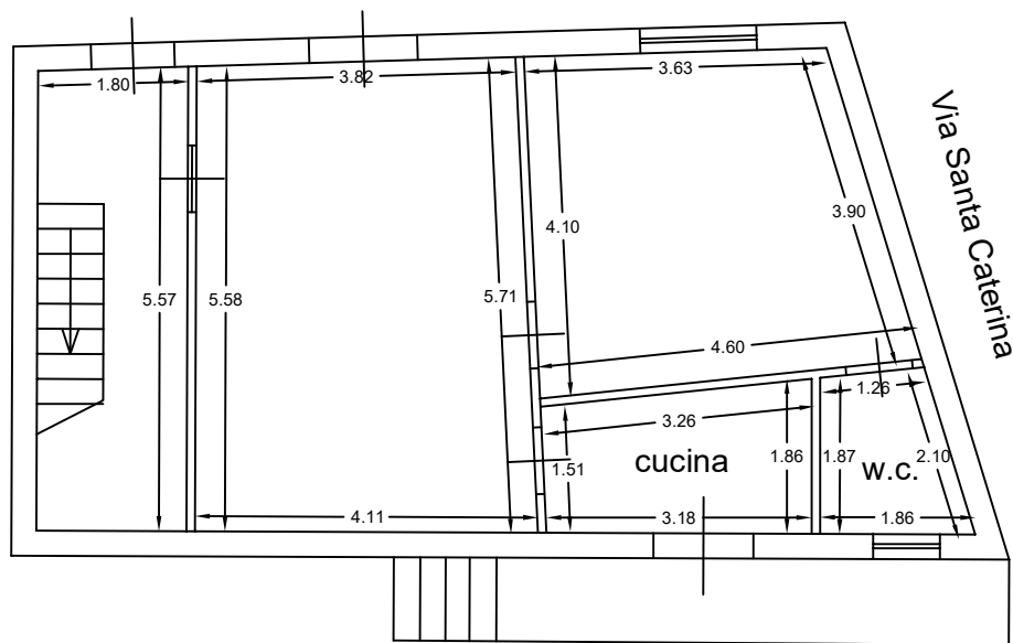
Pianta Piano Terra h= 3,50
