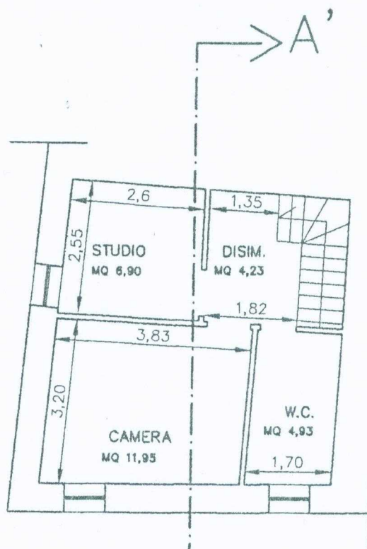
PIANTA PIANO SECONDO - Rapp. 1:100
