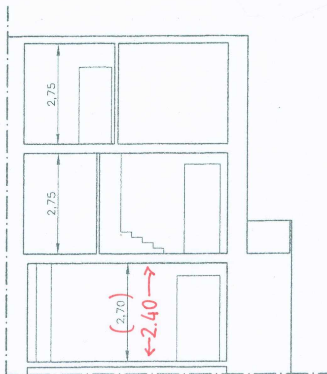
SEZIONE A-A'
