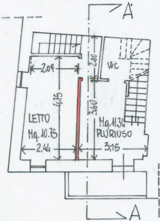
PIANTA PIANO PRIMO - 1:100
