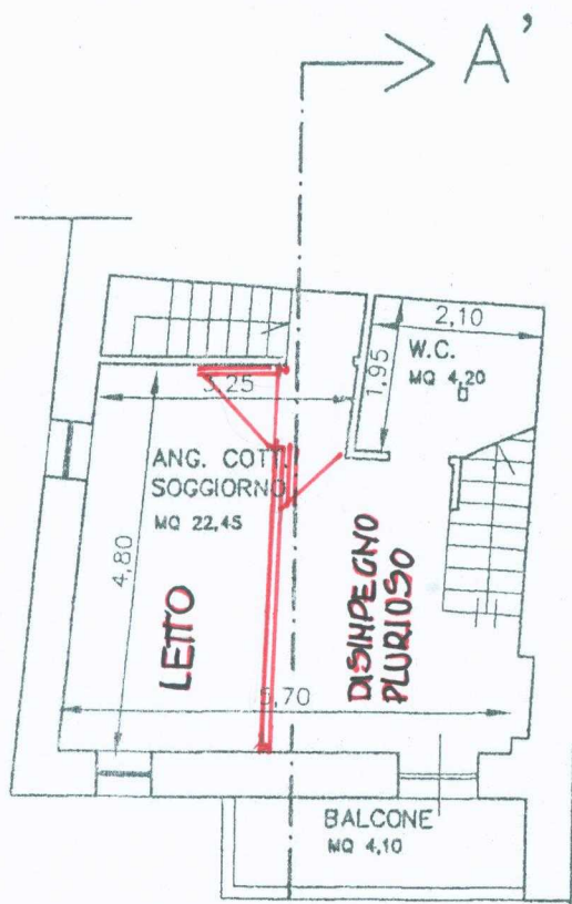
PIANTA PIANO PRIMO - Rapp. 1:100
