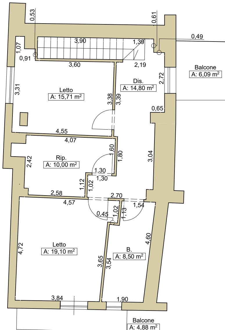
Pianta piano secondo - Fg. 9 P.IIa n. 670 - sub 18 - scala U
