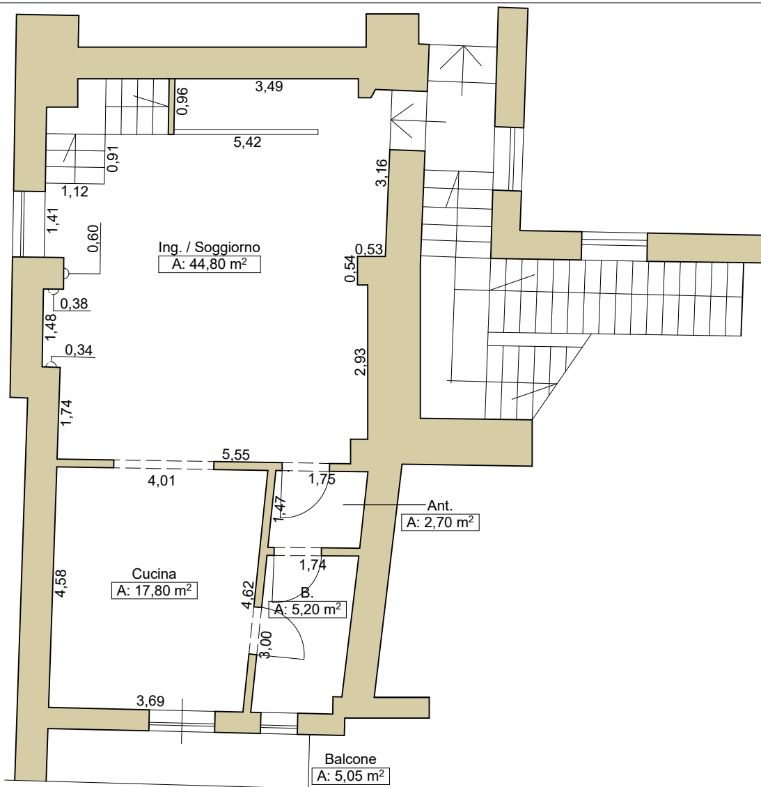
Pianta piano primo - Fg. 9 P.IIa n. 670 - sub 18 - scala U
