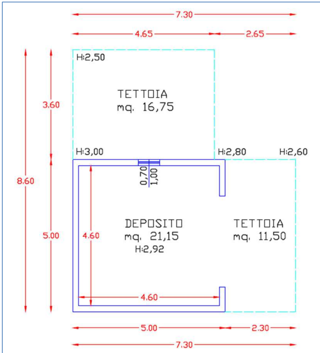
IMMAGINE 5- PLANIMETRIA FABBRICATO 1
