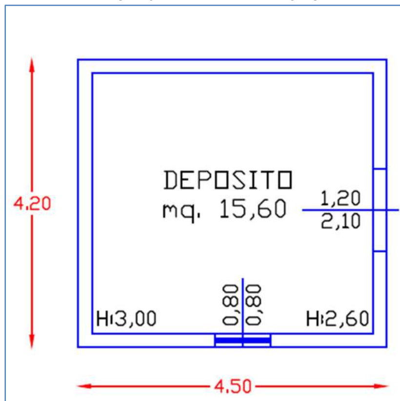
IMMAGINE 7- PLANIMETRIA FABBRICATO 3
