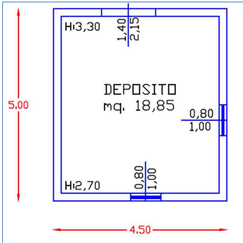
IMMAGINE 6- PLANIMETRIA FABBRICATO 2
