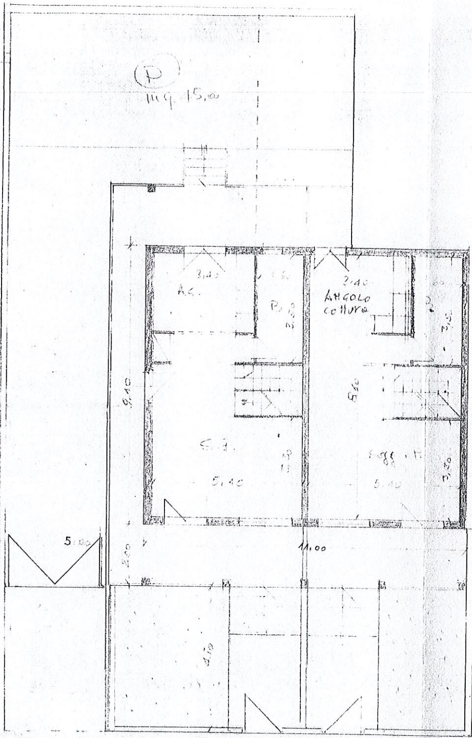
PIANTA PIANO TERRA 1:100
