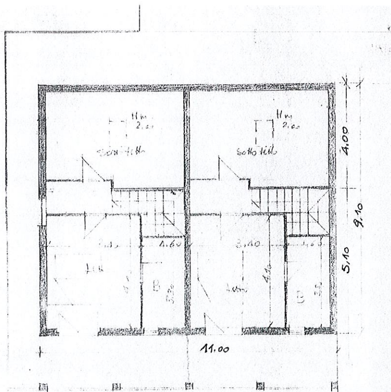
PIANTA PIANO PRIMO 1:100 VARIANTE
