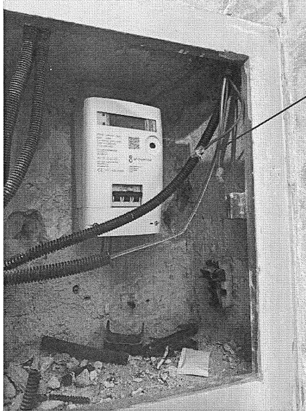
Foto 5 – Particolare del misuratore Enel posto all'ingresso del lotto "A"
