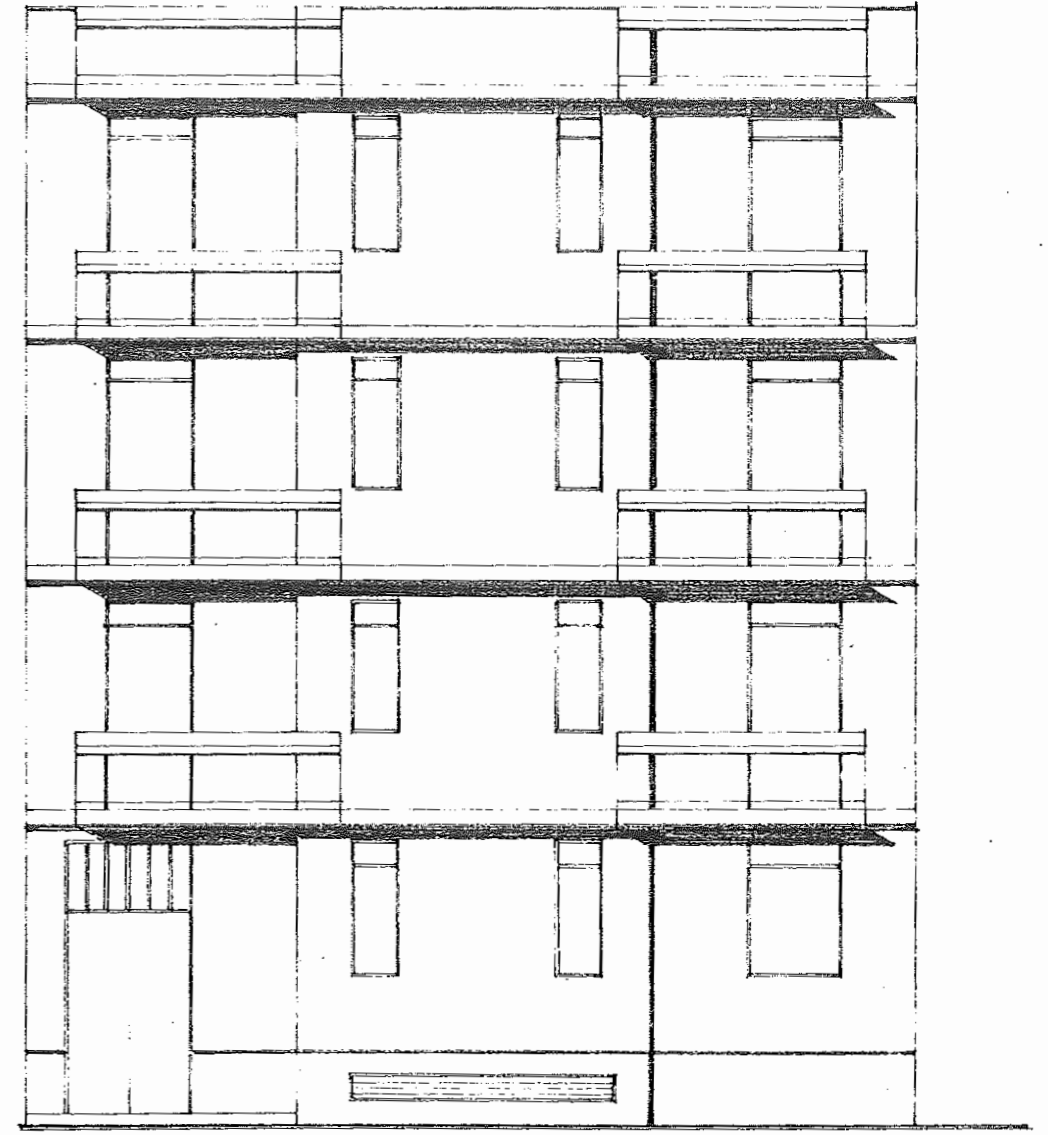
PROSPETTO VIA FONTENUOVO RAPP. 1/100
