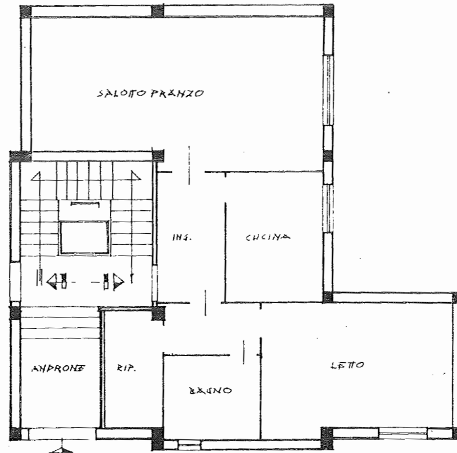
PIANTA PIANO RIALZATO
