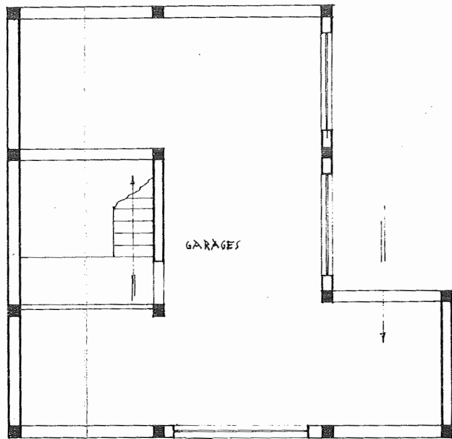
PIANTA PIANO INTERRATO
