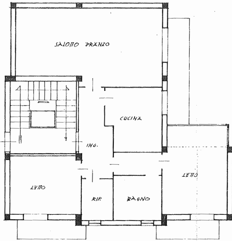
PIANTA PIANO TIPO RAPP. 1/100
