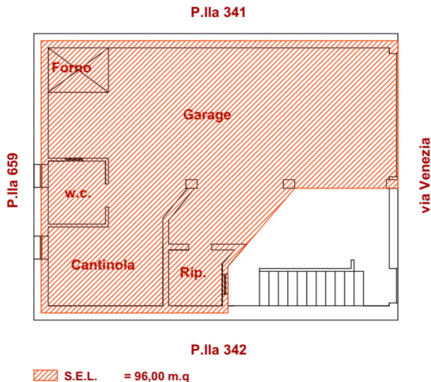
PLANIMETRIA INDIVIDUAZIONI SUPERFICI SUB 2
