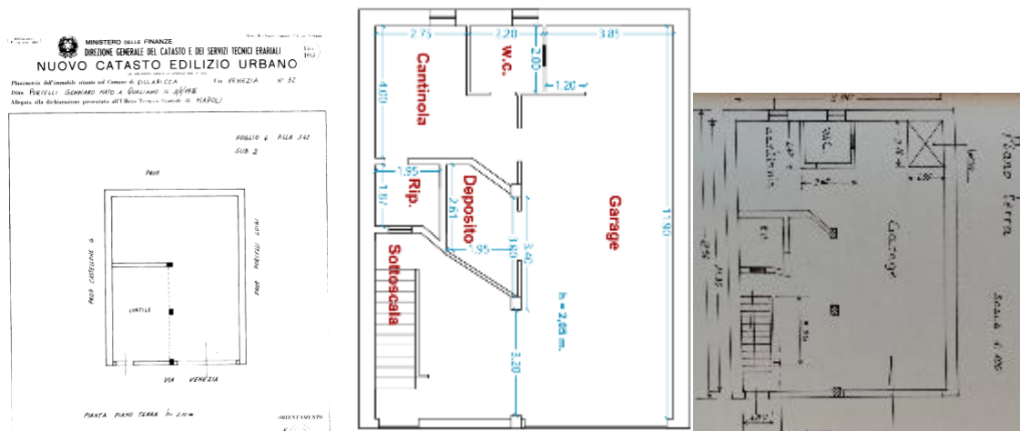
PLANIMETRIA STATO CATASTALE SUBALTERNO 2 PLANIMETRIA STATO ATTUALE SUBALTERNO 2 PLANIMETRIA DI CONDONO SUBALTERNO 2
