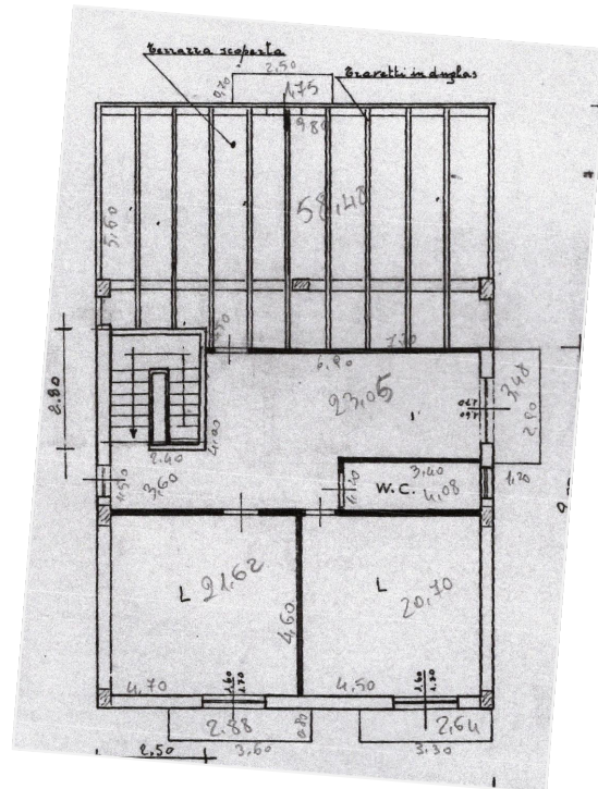
PIANTA PRIMO
