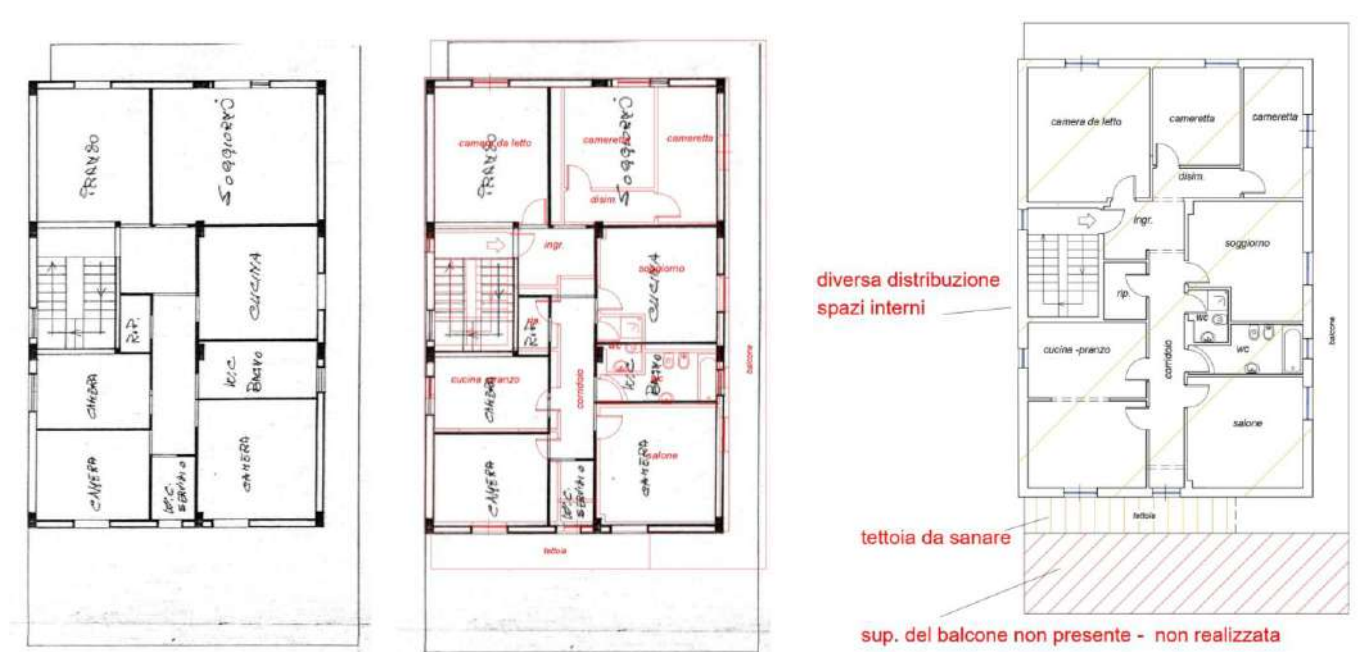
planimetria sanatoria
