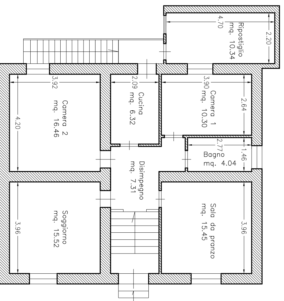
PIANTA PIANO RIALZATO scd1:100 STATO ATTUALE
