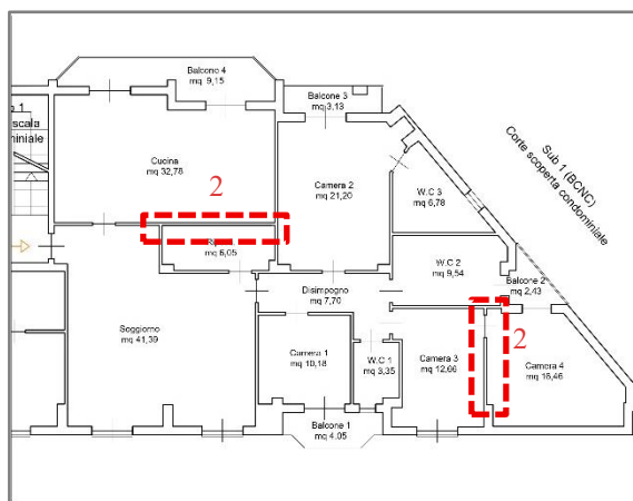
Pianta piano primo da rilievo geometrico effettuato durante il sopralluogo dal sottoscritto CTU
