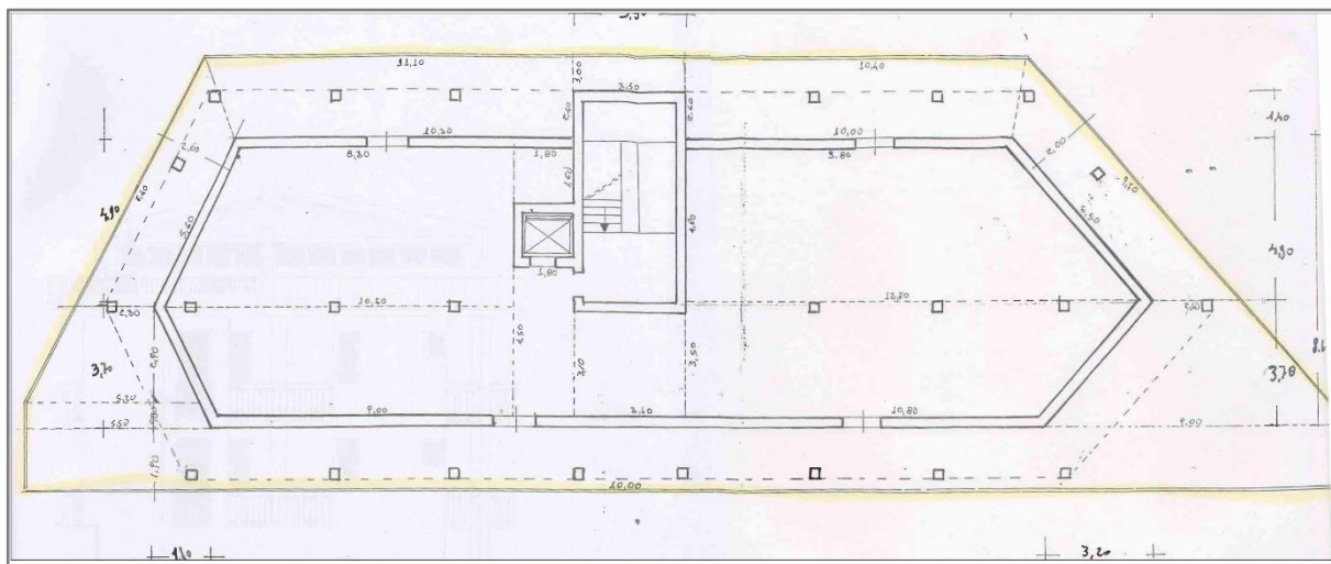
Pianta a corredo della Concessione Edilizia in sanatoria n. 81/2018 piano sottotetto terzo piano
