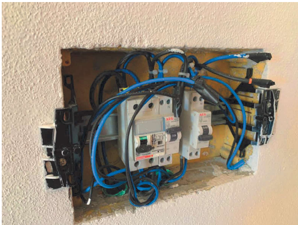
Foto n 9 Quadro elettrico
