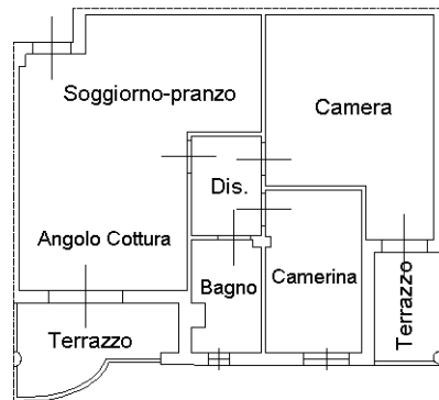
Piano Primo H= ml. 2,70
