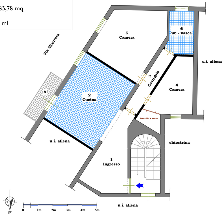
Planimetria di rilievo dello stato di fatto
