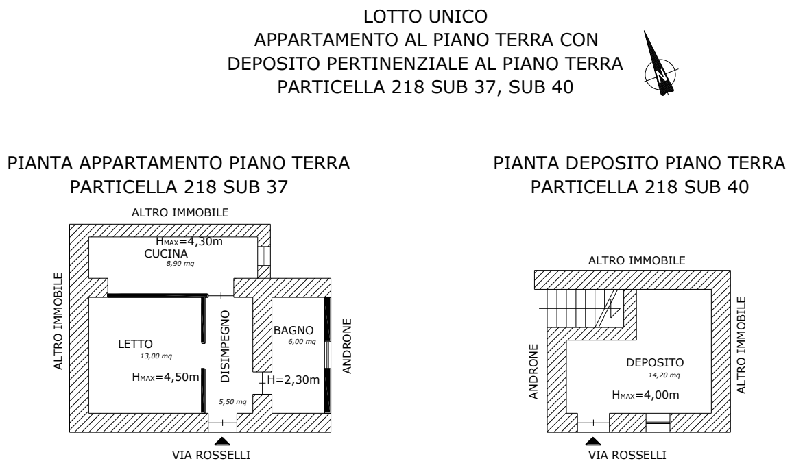
Figura 18 Planimetrie dell'appartamento al piano terra e del deposito pertinenziale al piano terra
