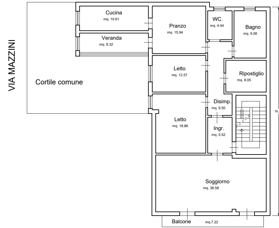
Pianta piano primo sc. 1:100 H. 3.00
