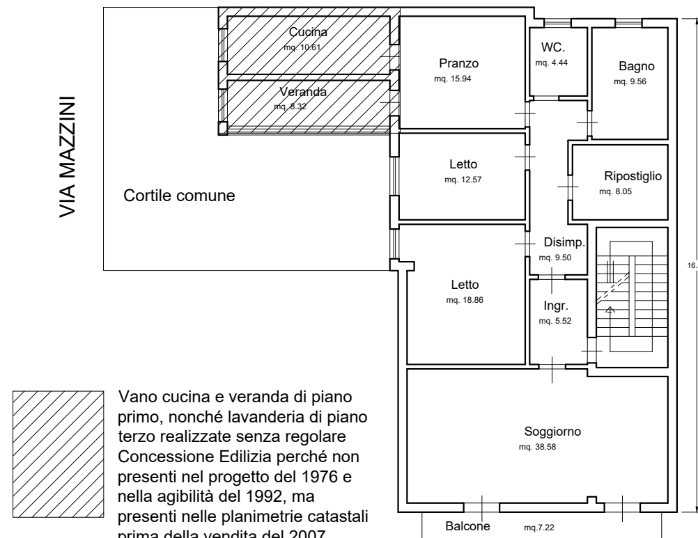
Pianta piano primo sc. 1:100 H. 3.00
