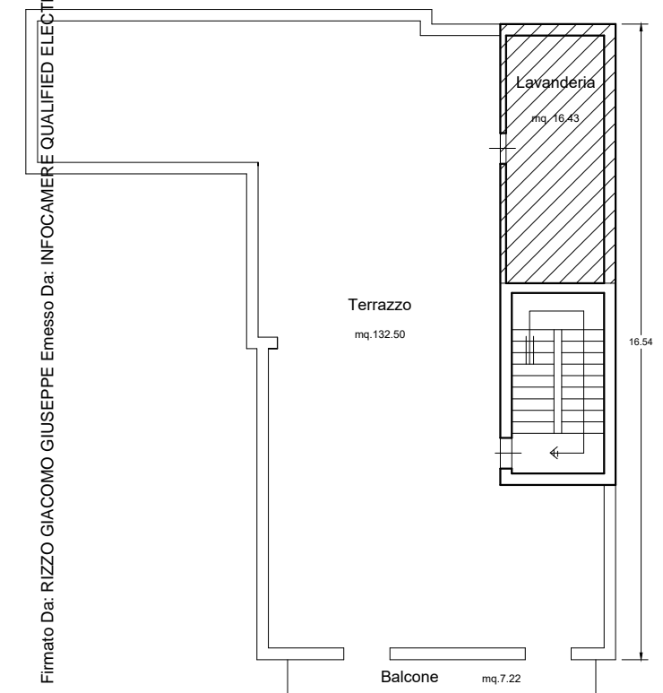
Pianta piano secondo sc. 1:100 H. 2.80
