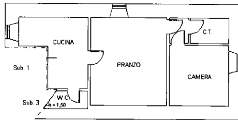
PIANTA PIANO TERRA h. 2,50 mt.
