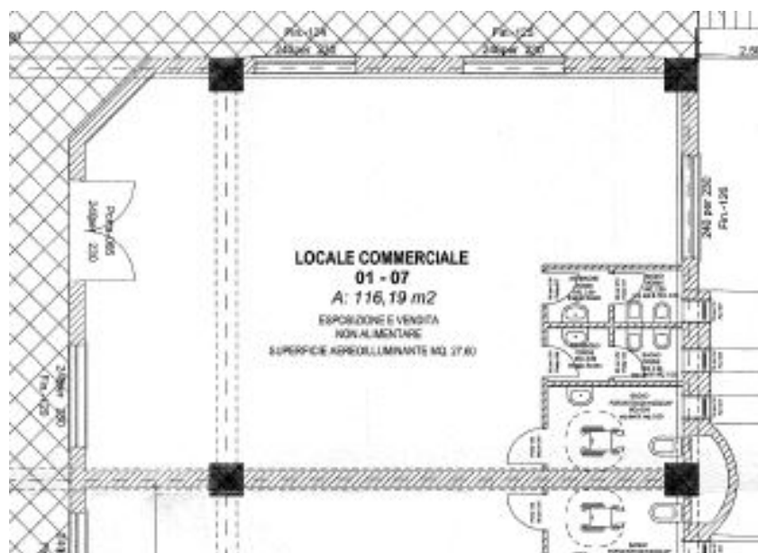
All. n. 15.3 – planimetria autorizzata
