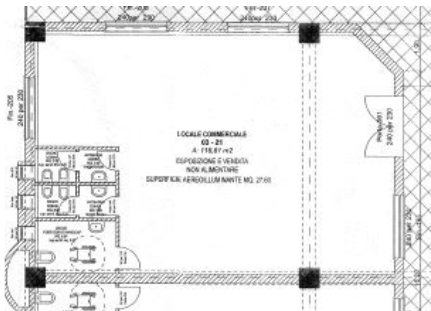
All. n. 15.16 – planimetria autorizzata
