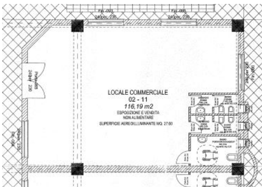
All. n. 15.6 – planimetria autorizzata
