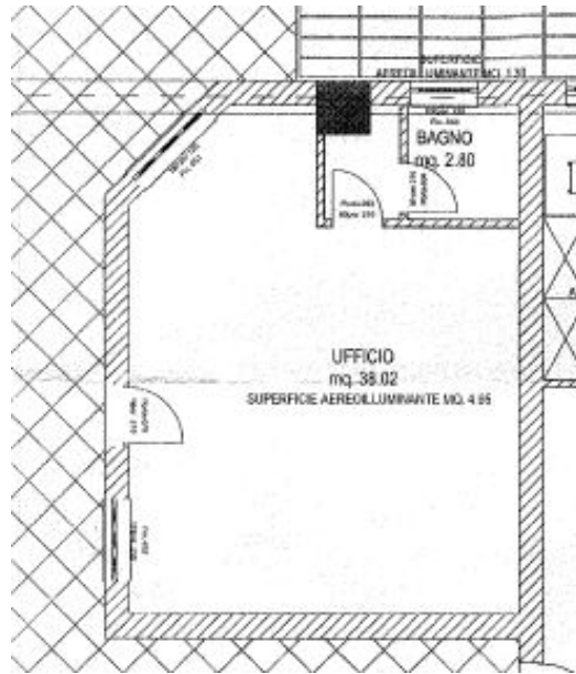
All. n. 15.9 – planimetria autorizzata
