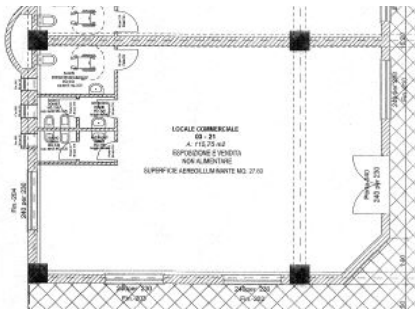
All. n. 15.15 – planimetria autorizzata
