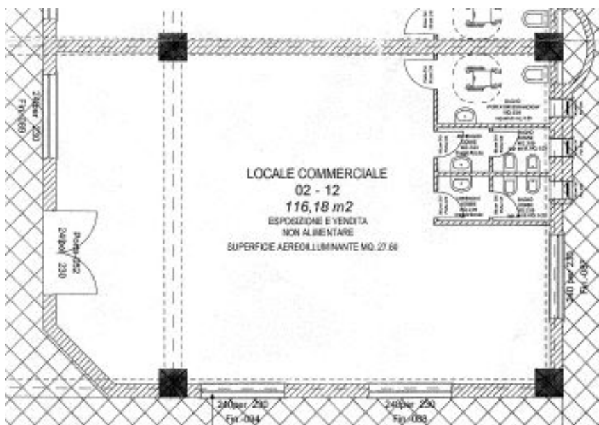
All. n. 15.5 – planimetria autorizzata
