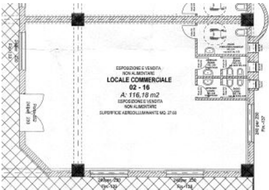
All. n. 15.8 – planimetria autorizzata
