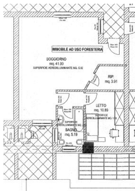
All. n. 15.12 – planimetria autorizzata
