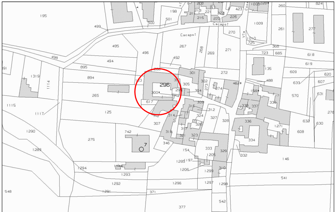
STRALCIO CATASTALE
