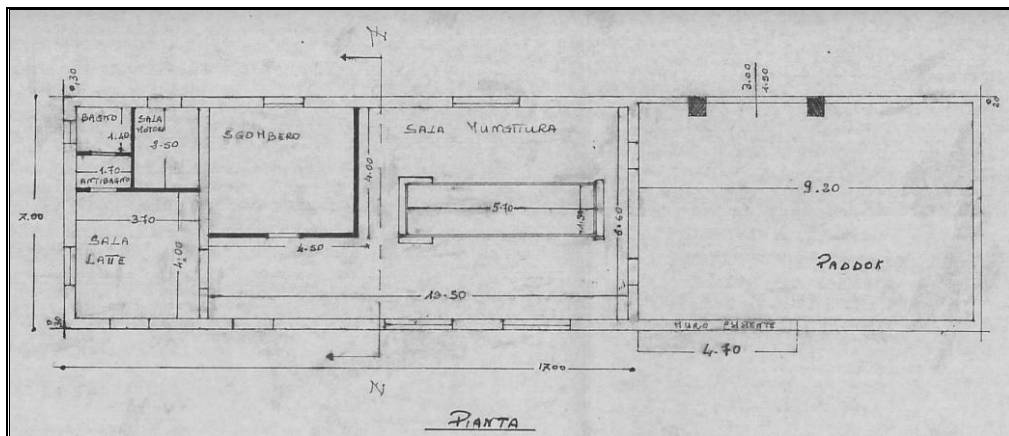
Immagine 5-Piano Terra
