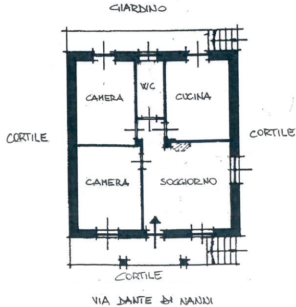
PIANTA PIANO TERRENO-RIALZATO
