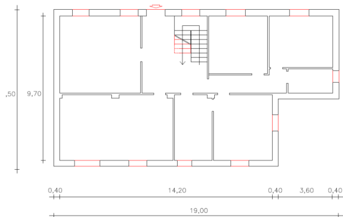
Pianta Piano Primo h= 2,85 mt
