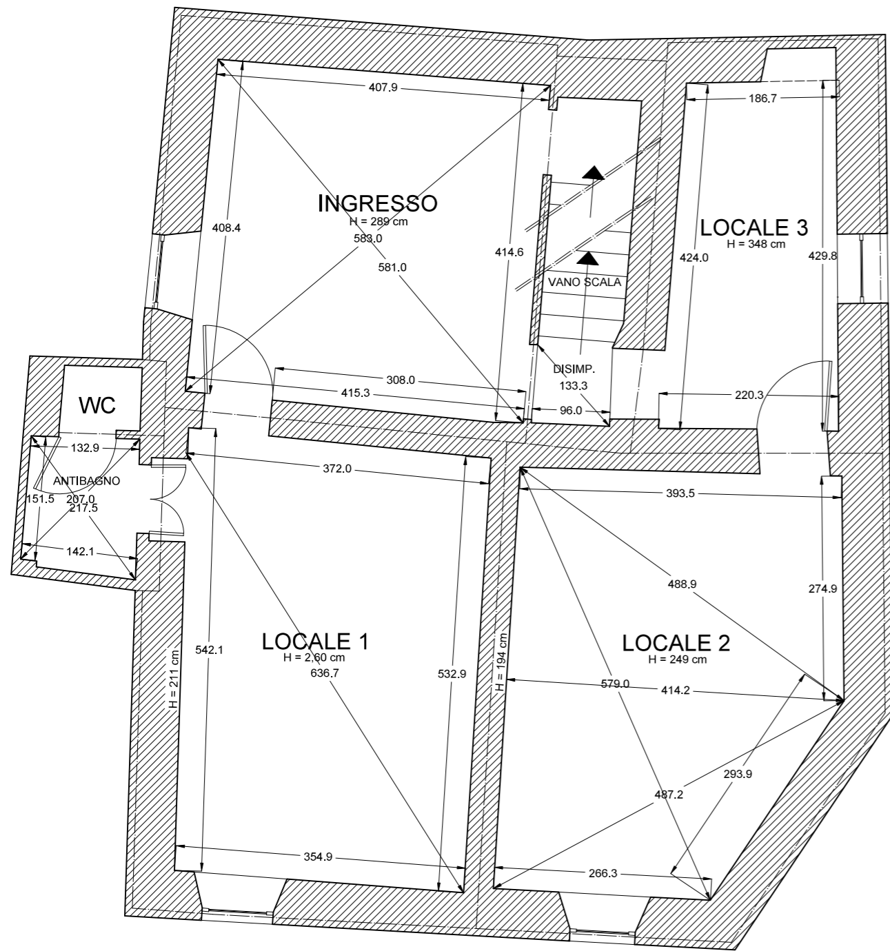
PIANTA TERZO MAPP. 210 SUB.11 - MAPP. 212 SUB. 9
