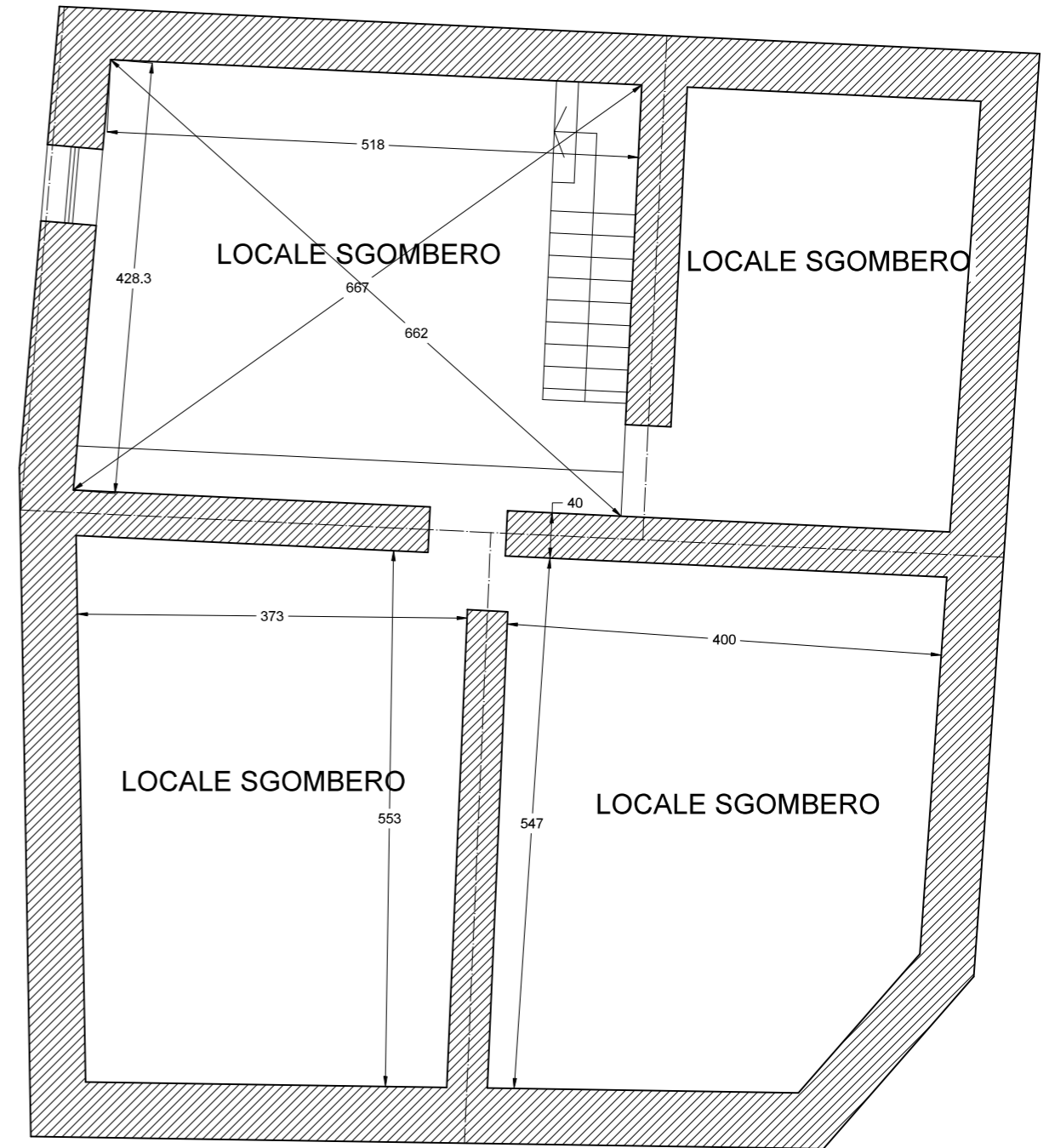
PIANTA TERZO MAPP. 210 SUB.11 - MAPP. 212 SUB. 9
