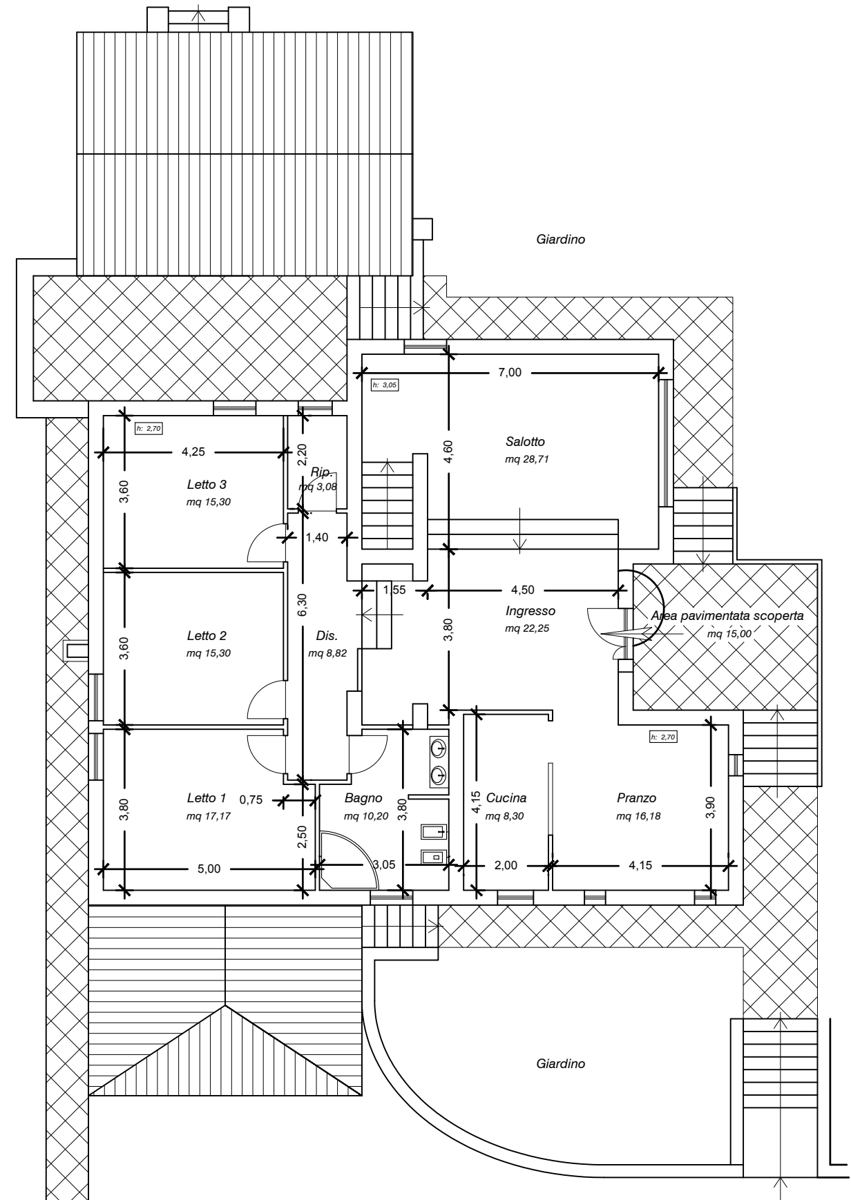
PIANTA PIANO FUORI TERRA
