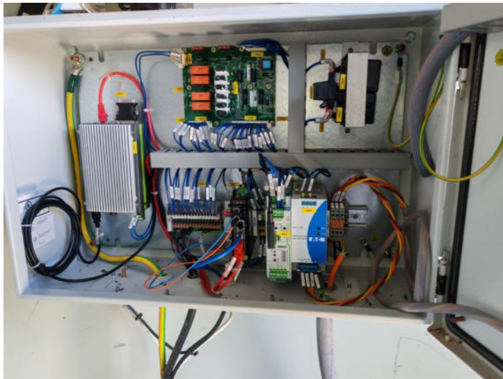
Foto n. 25 – Vista pala eolica – componenti interni
