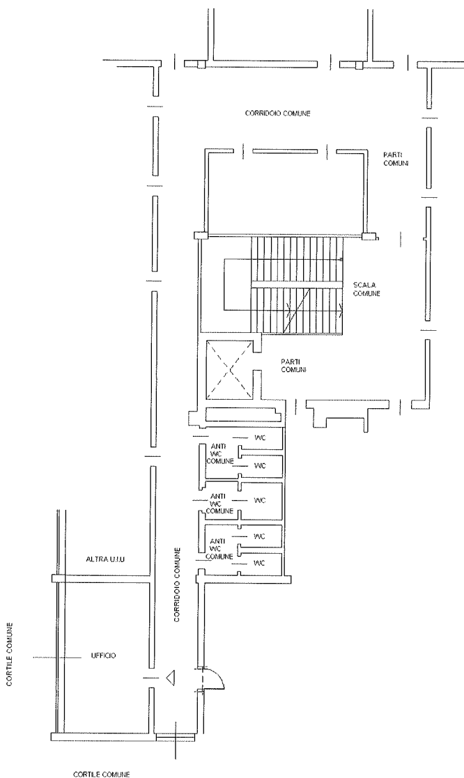
PIANO SECONDO H=4.45
