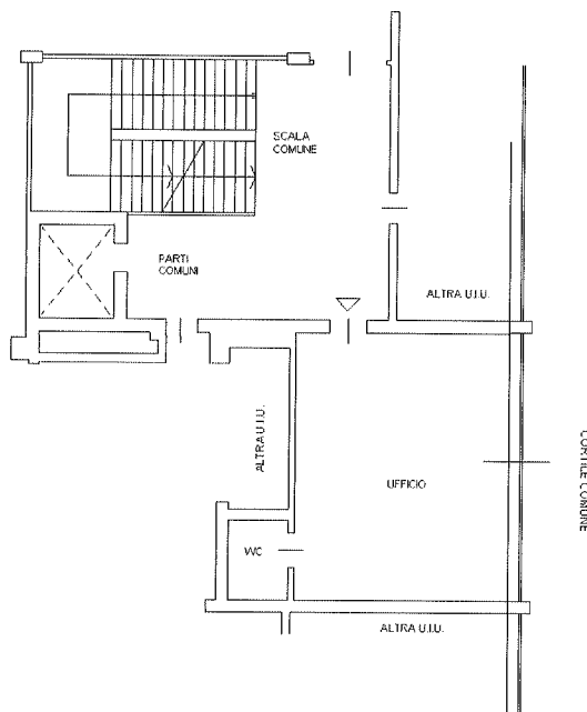
PIANO SECONDO H=4.45
