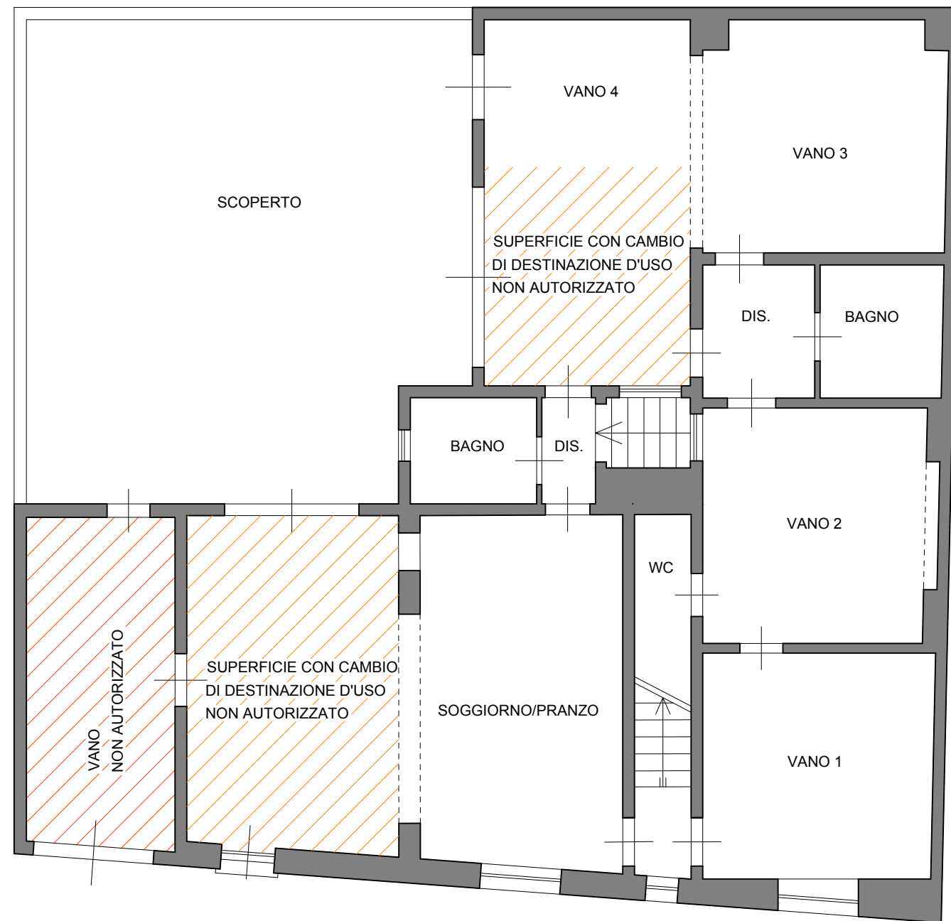
PIANTA PIANO TERRA - STATO DI FATTO RAPP. 1:100
