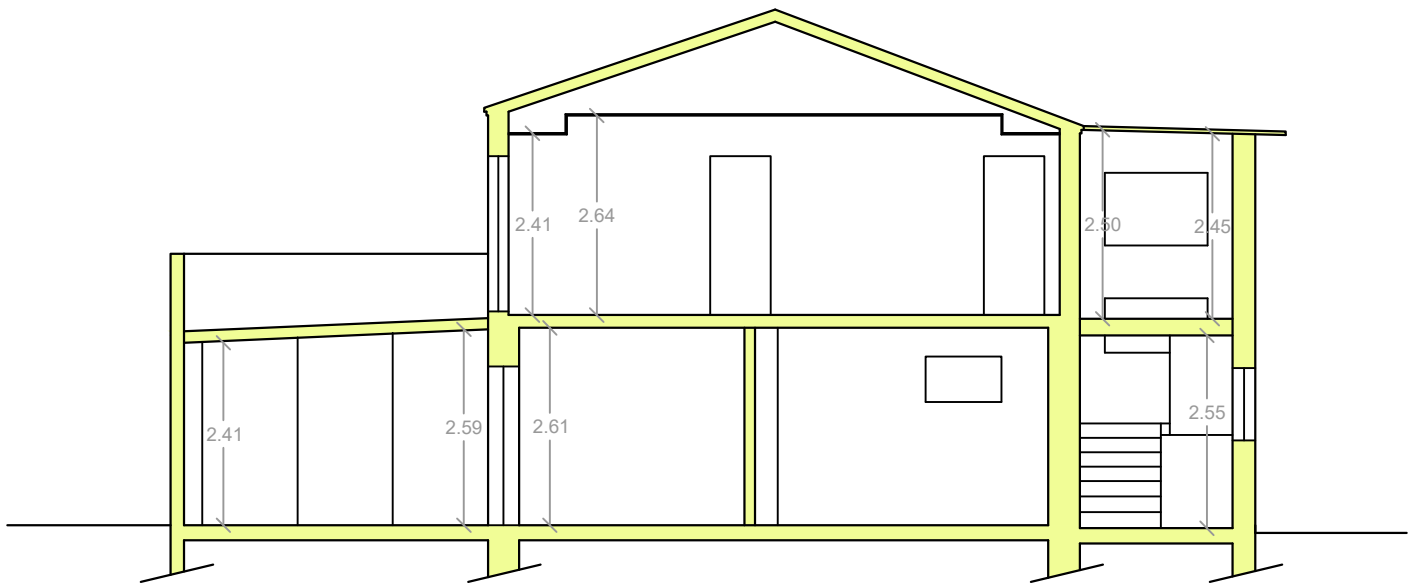
Sezione A-A'
