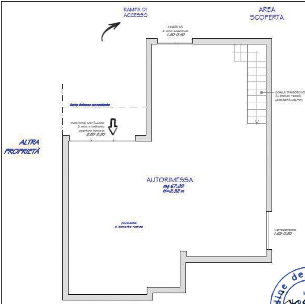
PIANTA GARAGE
