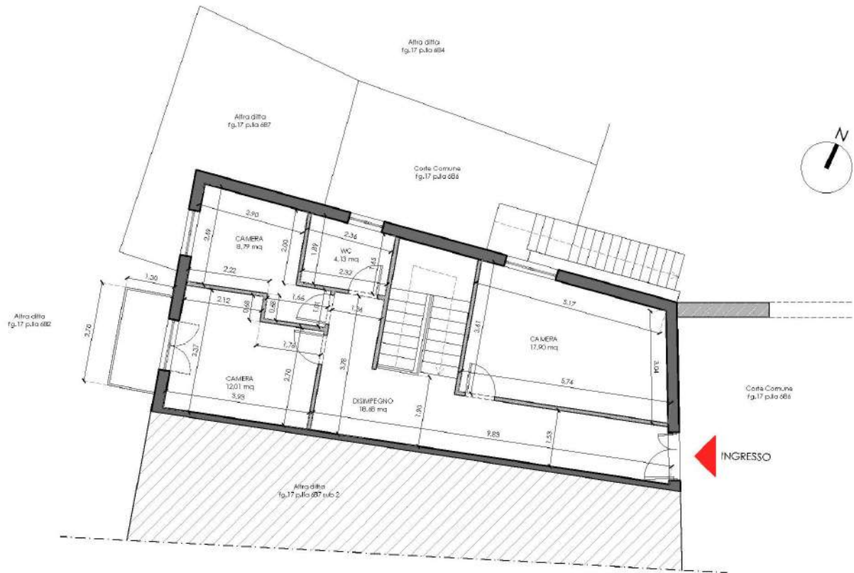
Figura 9: Rilievo Lotto Unico Stato di fatto _ pianta piano terra (Allegato 6E)
