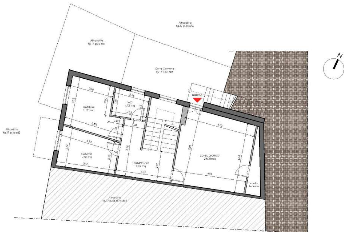
Figura 8: Rilievo Lotto Unico Stato di fatto _ pianta piano seminterrato (Allegato 6E)
