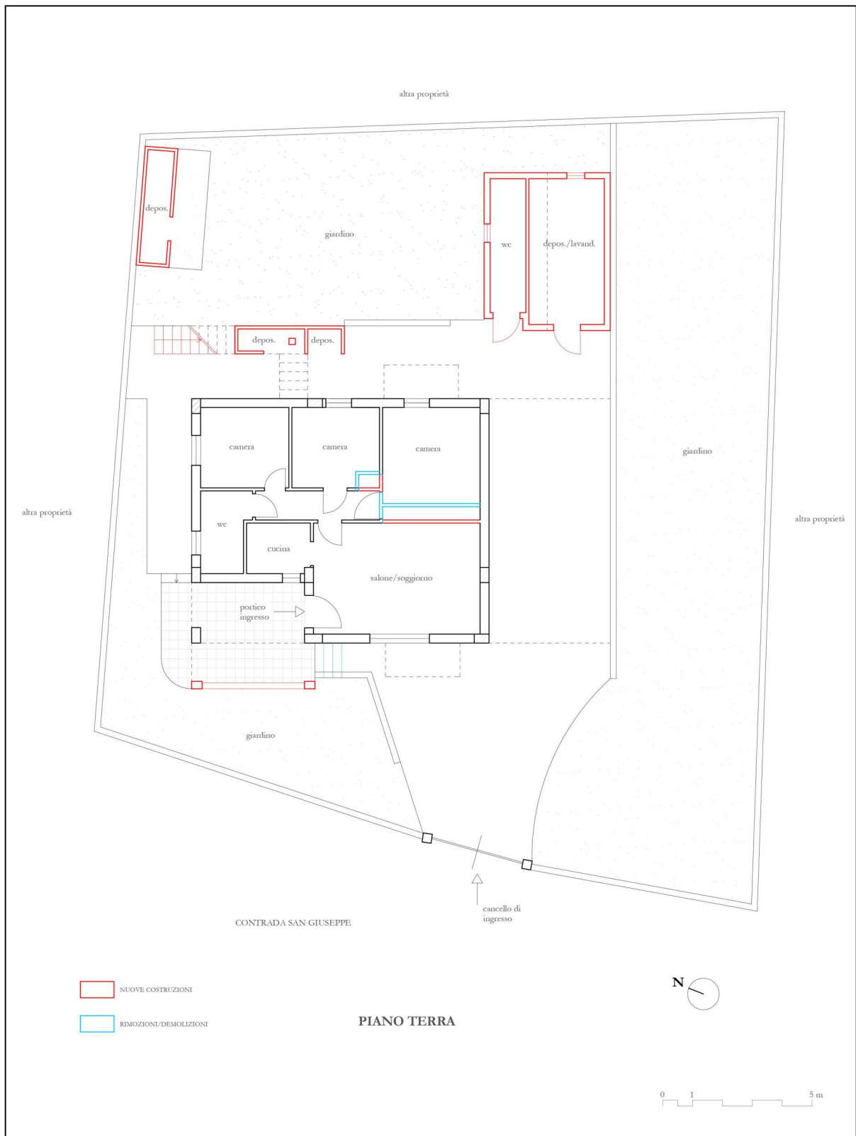
Rilievo attuale dei luoghi con indicazione grafica delle difformità riscontrate rispetto alla planimetria catastale. Piano terra (All. 16)
