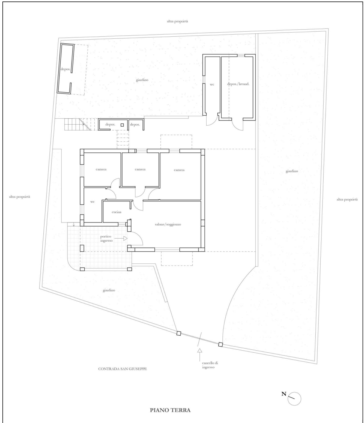
Planimetria di rilievo dello stato di fatto. Planimetria generale, piano terra (All. 15)
