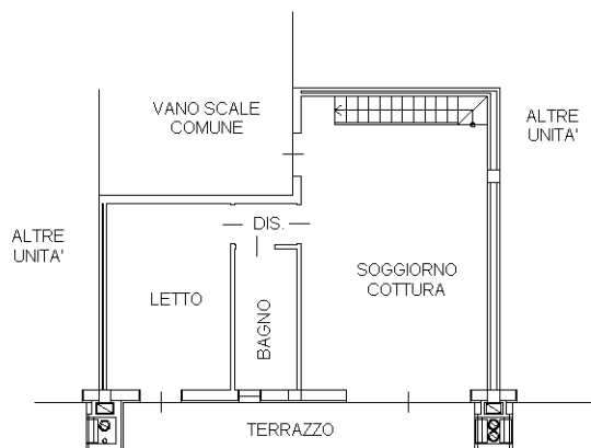
PIANTA PIANO SECONDO H = 2.70
