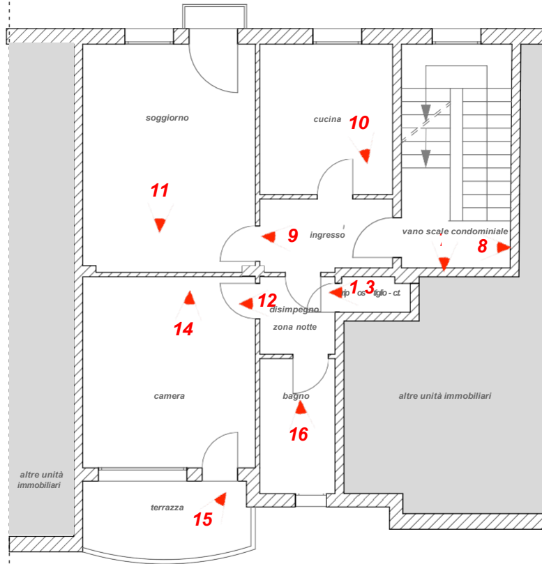
PIANO PRIMO H = 2,77
