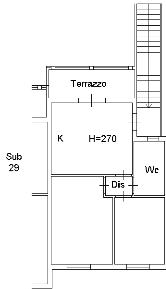
PIANO PRIMO
