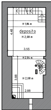
Pianta Piano INTERRATO
