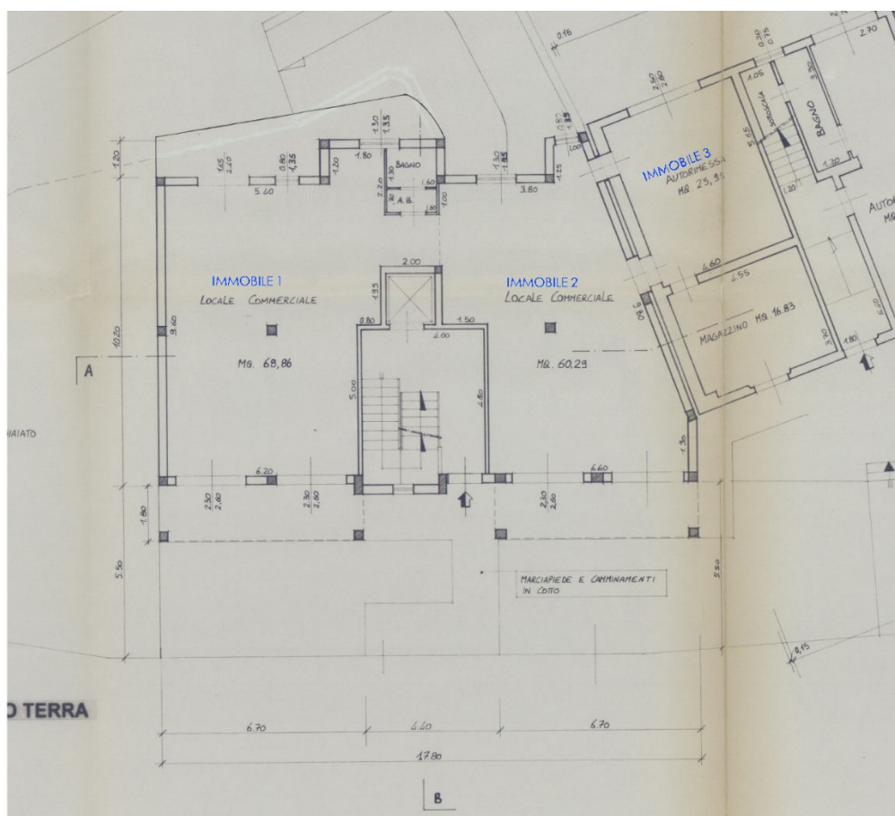
Figura 1 – planimetria dello stato legittimo
