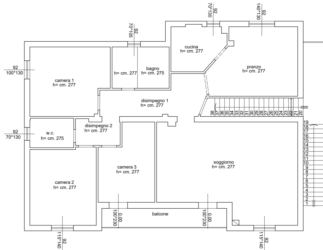
PIANTA PIANO SECONDO RAPP. 1:100
