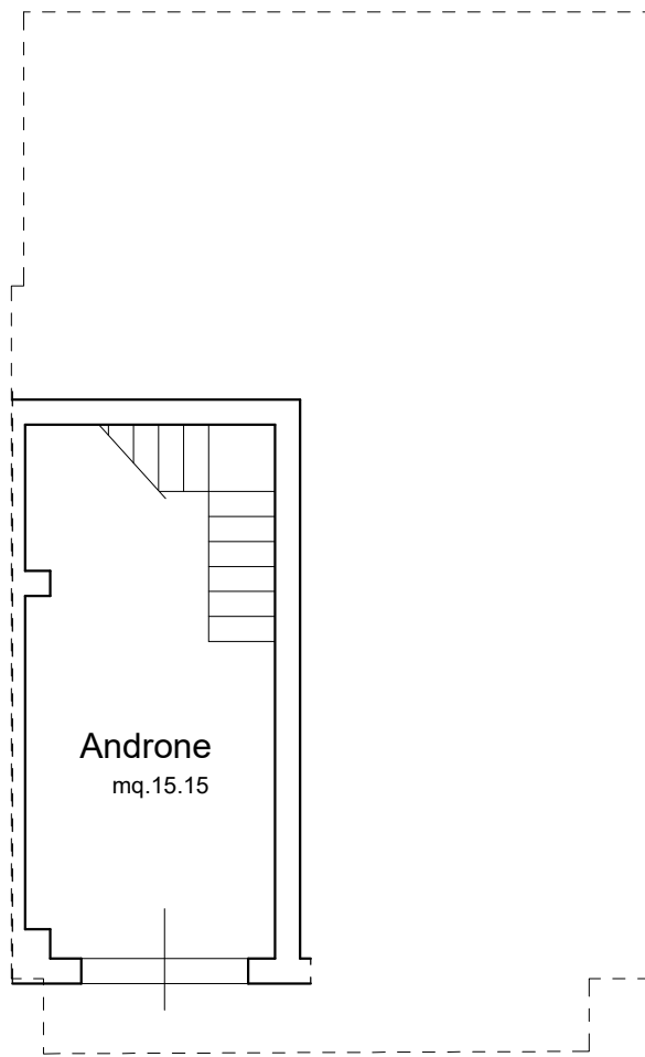
Pianta piano terra sc. 1:100
