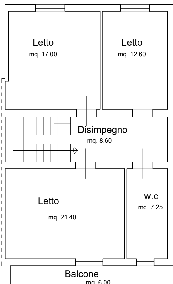
Pianta piano secondo sc. 1:100
