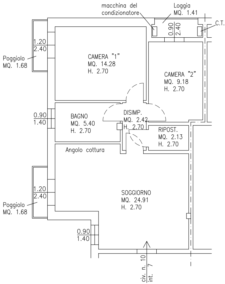
PIANO PRIMO
