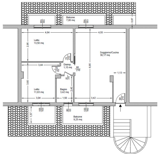
Planimetria Stato dei Luoghi
