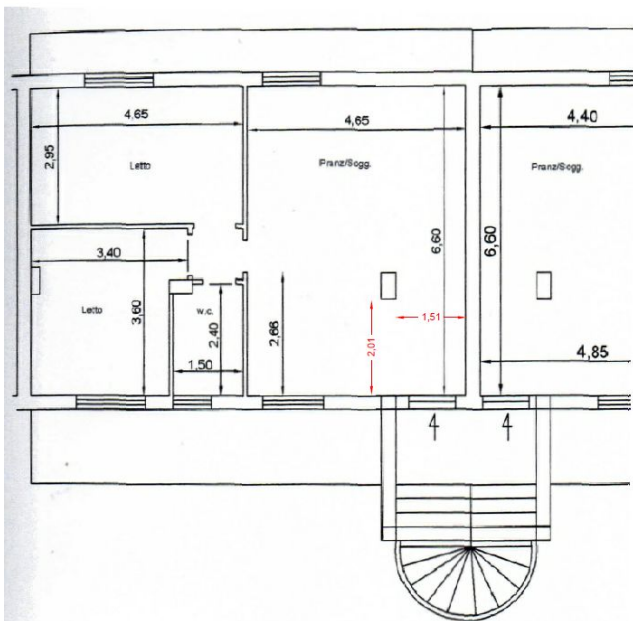
Planimetria di Progetto DIA prot. n. 2023 del 22/03/2006
