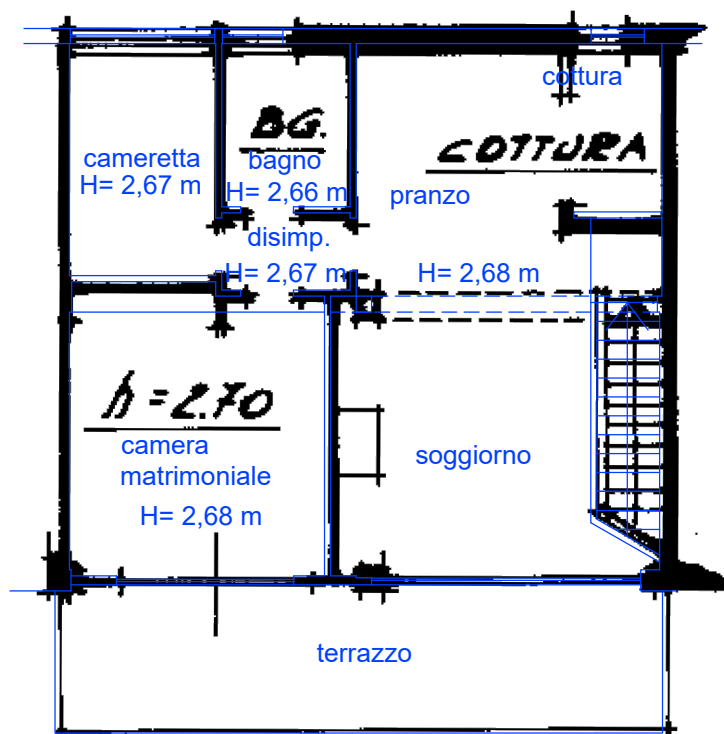
secondo livello - scala 1:100
