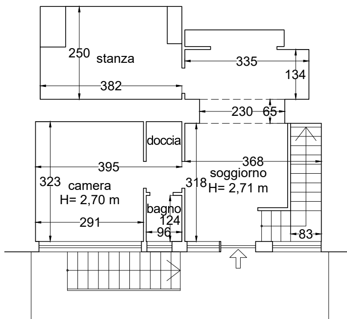
primo livello - scala 1:100
