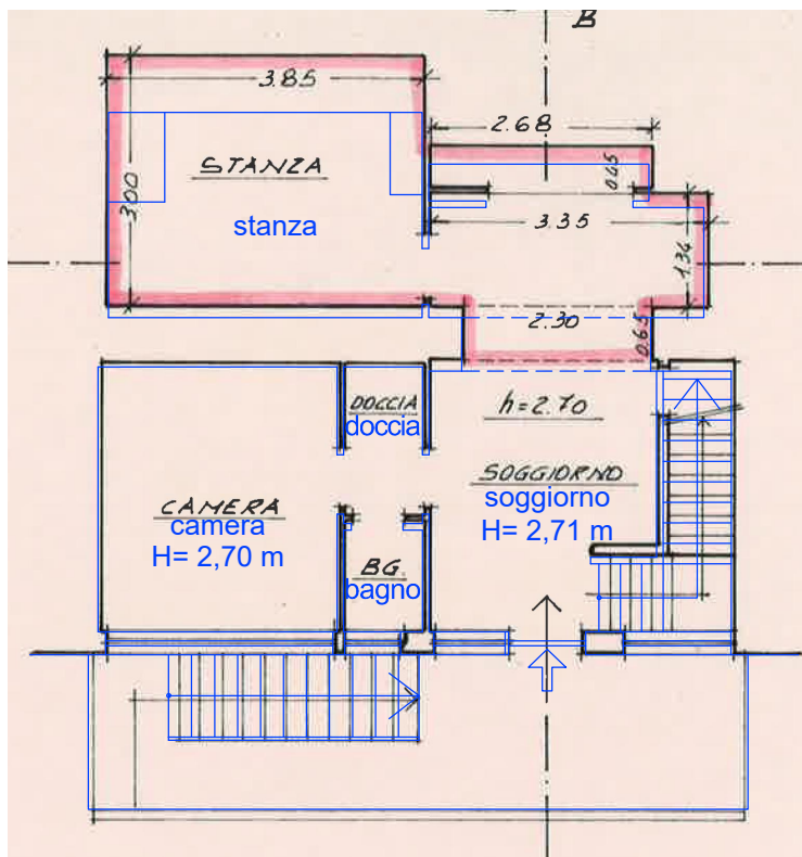
primo livello - scala 1:100
