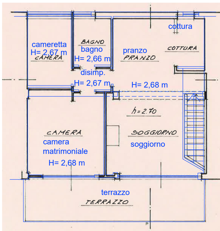
secondo livello - scala 1:100
