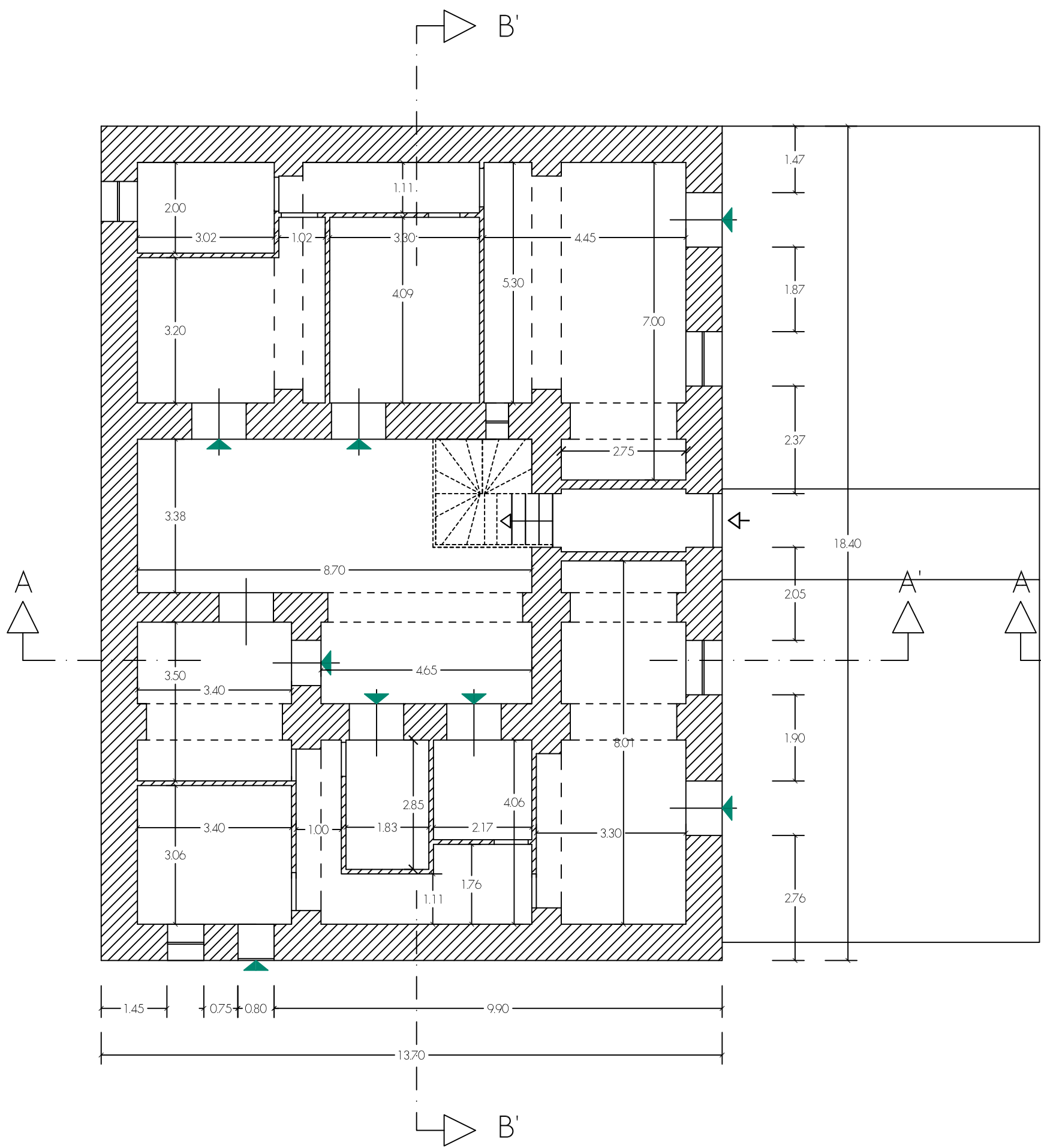
SEZIONE AA'
