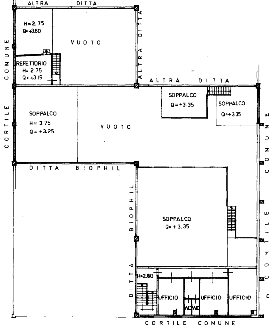
PIANO PRIMO
