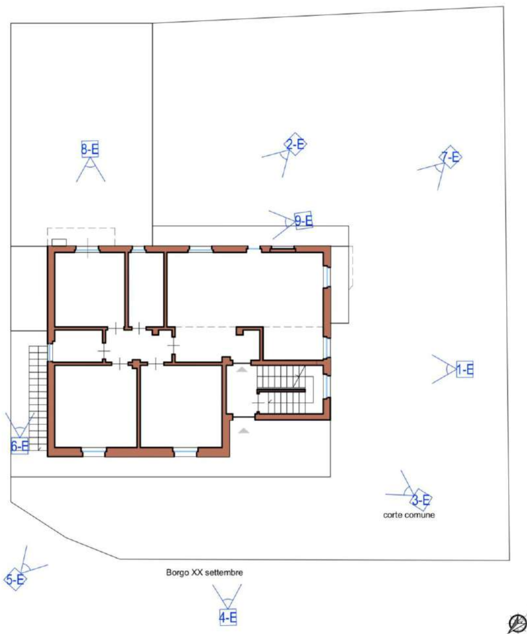
Pianta piano terra con coni ottici esterni
