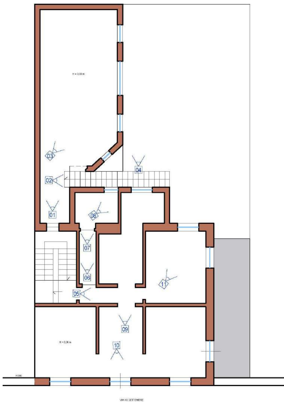
Pianta piano primo con coni ottici
