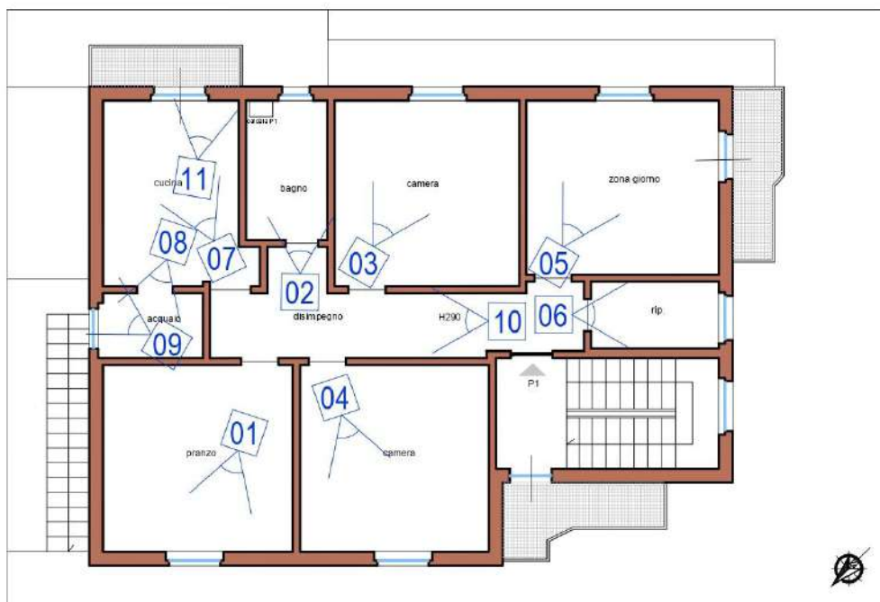
Pianta piano primo con coni ottici
