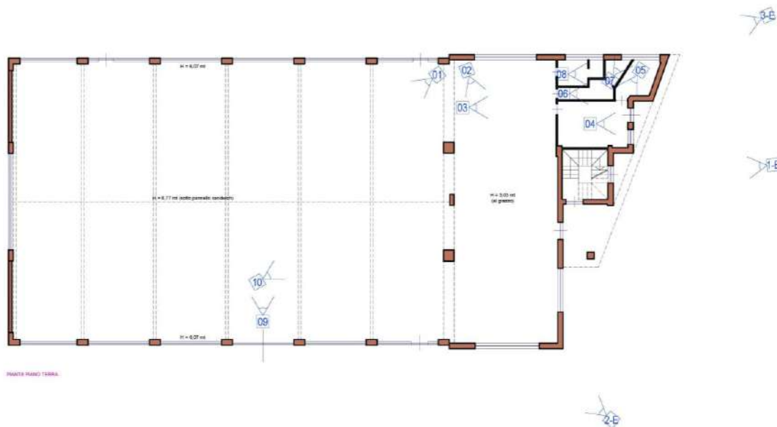
Pianta piano terra con coni ottici interni ed esterni
