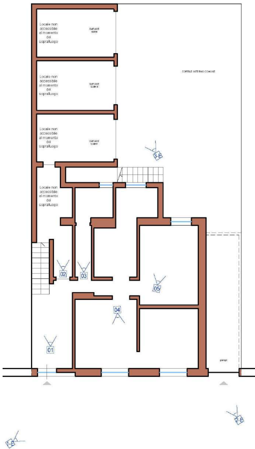
Pianta piano terra con coni ottici interni ed esterni
