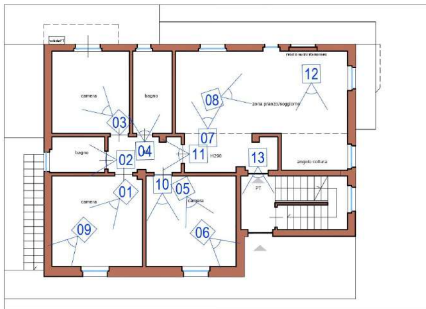
Pianta piano terra con coni ottici
