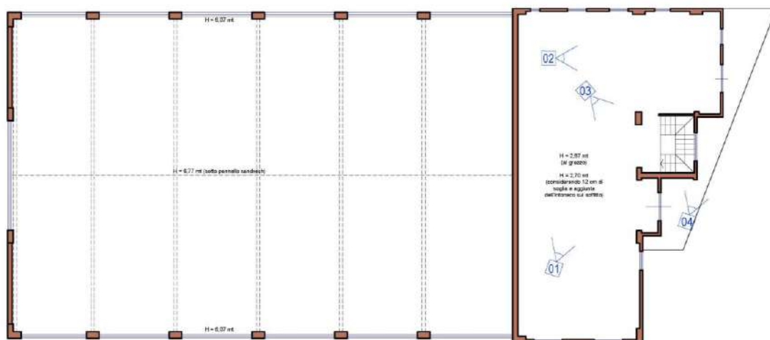
Pianta piano primo con coni ottici
