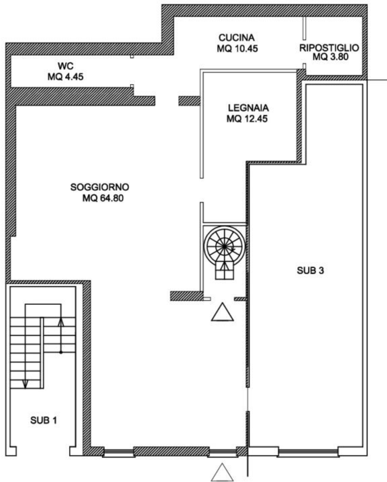
PIANTA APPARTAMENTO A – STATO ATTUALE – PIANO SEMINTERRATO
